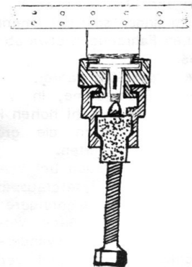
Lager abziehen:
